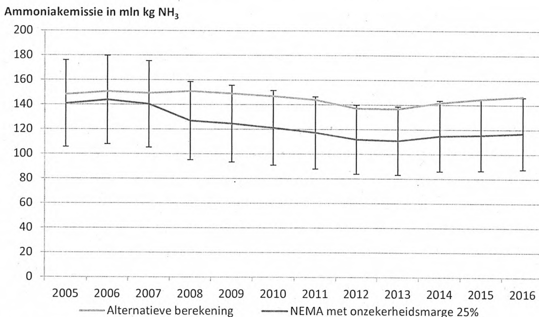
Figuur B6. Ammoniakemissie met aannames voor emissiearme huisvesting, export en mestverwerking (verbranding/kalvergierzuivering) en mesttoediening (miljoen kg \text{NH}_3 ).
