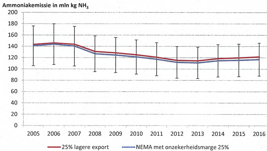
Figuur B4. Ammoniakemissie bij 25% lagere mestexport (miljoen kg NH 3 ). De niet-geëxporteerde mest wordt aan landbouwgronden in Nederland toegediend.
