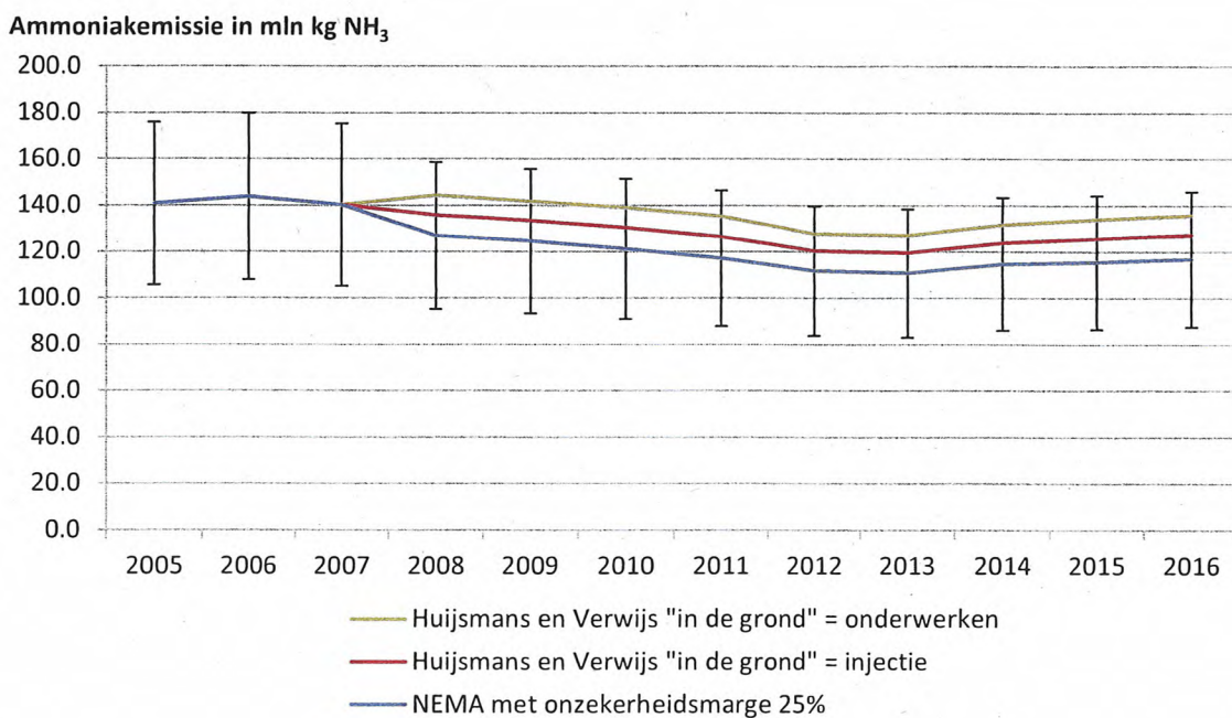
Figuur B5. Ammoniakemissie met aangepaste implementatiegraden van werkresultaten (miljoen kg NH 3 ). In de analyse is uitgegaan van de implementatiegraden op grasland en bouwland uit Huijsmans en Verwijs (2008) waarbij voor bouwland is uitgegaan dat het aandeel "in de grond" in één scenario volledig is toegerekend aan injectie en één keer volledig aan inwerken. Over de periode vóór 2008 is geen informatie beschikbaar over werkresultaten in de praktijk.
