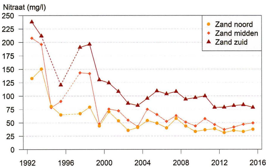
Figuur 2. Nitraatconcentraties (als \text{NO}_3 in mg per liter) in het water dat uitspoelt uit de wortelzone op landbouwbedrijven voor de drie zandgebieden in de periode 1992-2015. Jaargemiddelden van gemeten concentraties (Fraters et al., 2016).
