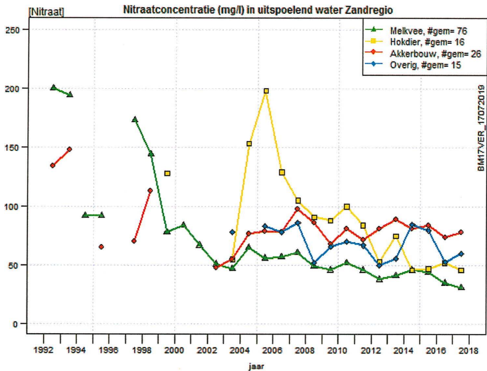
Figuur 3. Nitraatconcentraties (als \text{NO}_3 in mg per liter) in het water dat uitspoelt uit de wortelzone op verschillende typen landbouwbedrijven in de Zandregio in de periode 1992-2014. Jaargemiddelden van gemeten concentraties. Bron: LMM.
