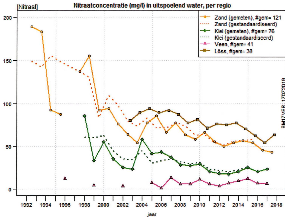
Figuur 1. Nitraatconcentraties (als \text{NO}_3 in mg per liter) in het water dat uitspoelt uit de wortelzone op landbouwbedrijven per regio in de periode 1992-2017. Jaargemiddelden van gemeten concentraties (Bron: LMM).
