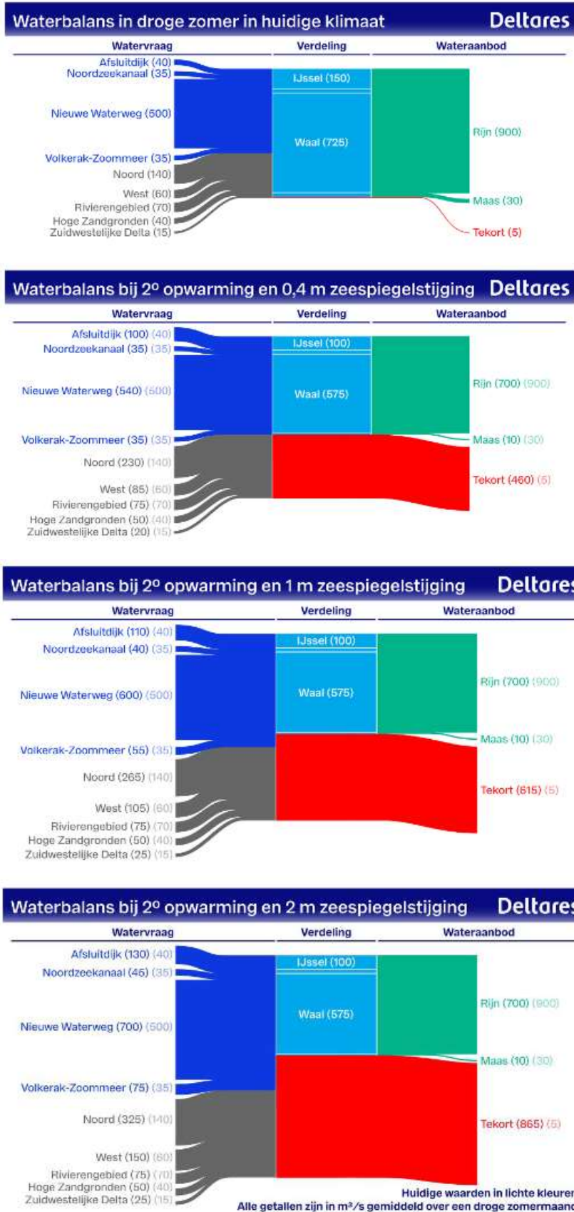
Figuur 6 Waterbalansen laag-Nederland
