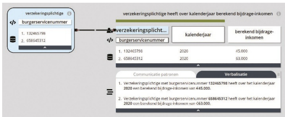
Figuur 6.13 Schermafbeelding feitmodel in iKnow Data
