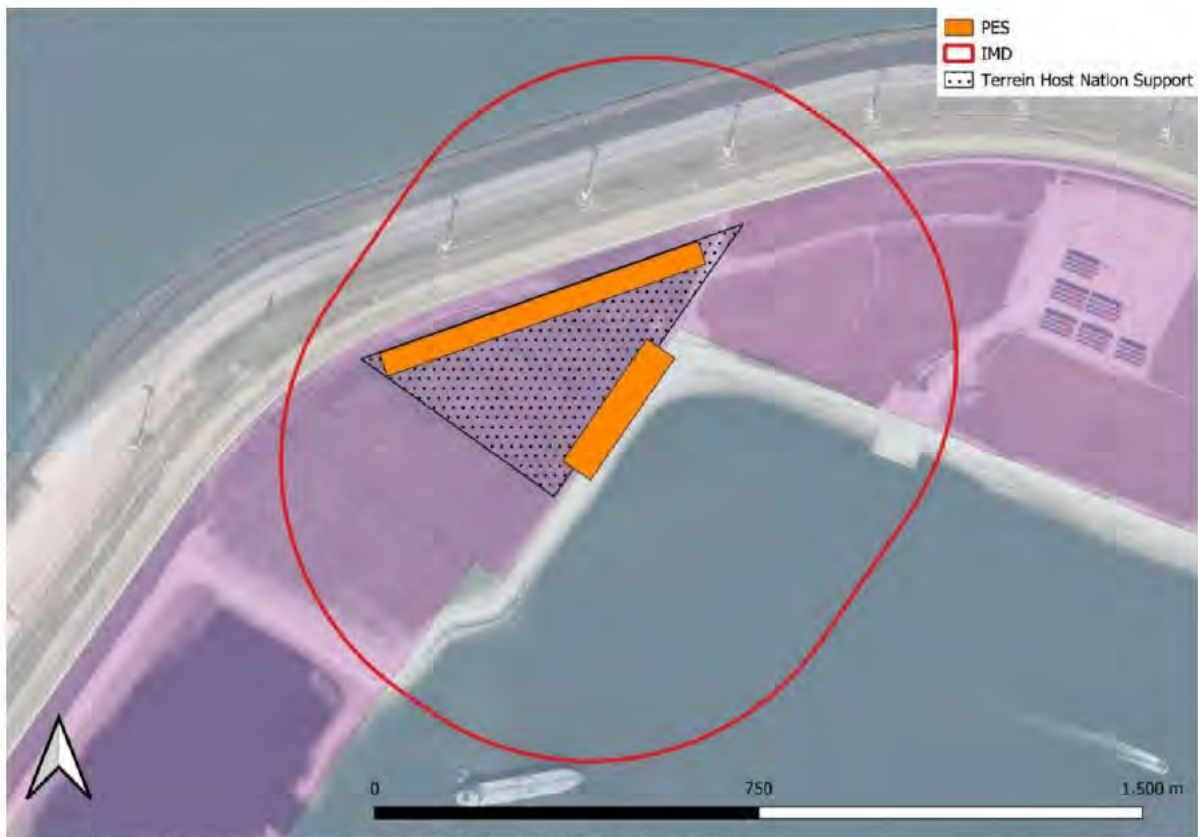
figuur 3-23 Overslaglocatie met inwendige veiligheidsafstand (IMD). Bron: TNO 2026
