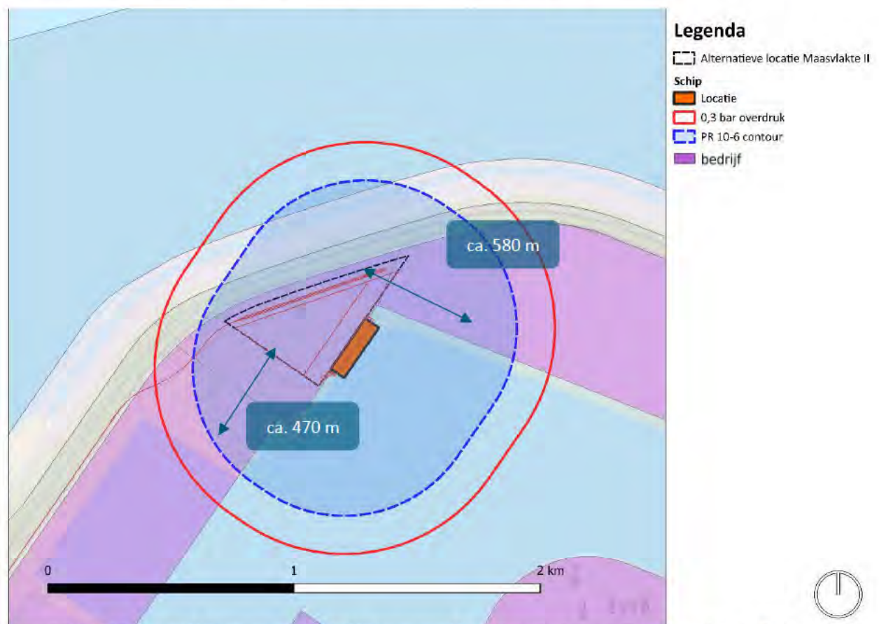
figuur 3-20 De 0,3 bar overdruk contour en de PR 10^{-6} -contour van het schip op basis van voorgaande onderzoek: Resultaten QRA Defensierrein RWG v2 (TNO, 2025). Daarnaast is de enkelbestemming bedrijf weergegeven.
