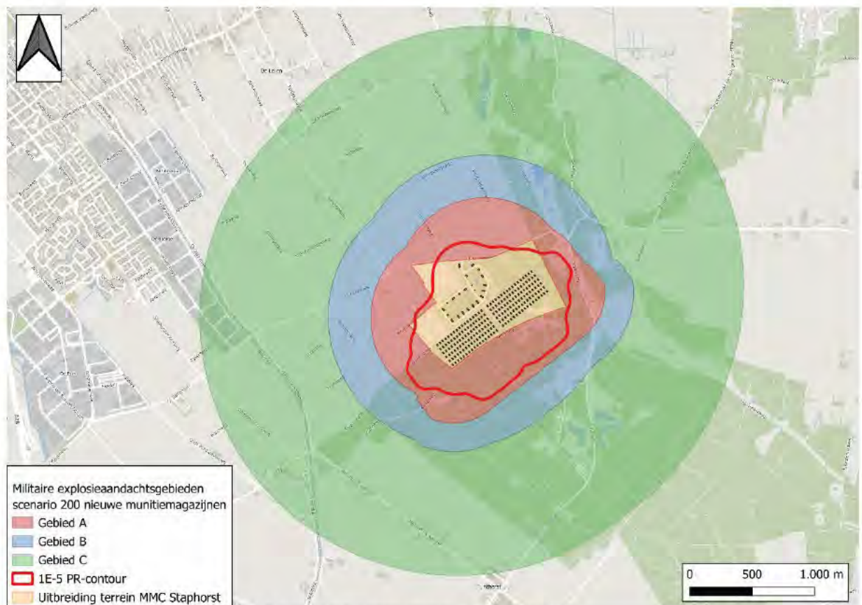
figuur 3-11 Berekening van de 10^{-5} /jaar plaatsgebonden risicocontouren in de nieuwe situatie.
