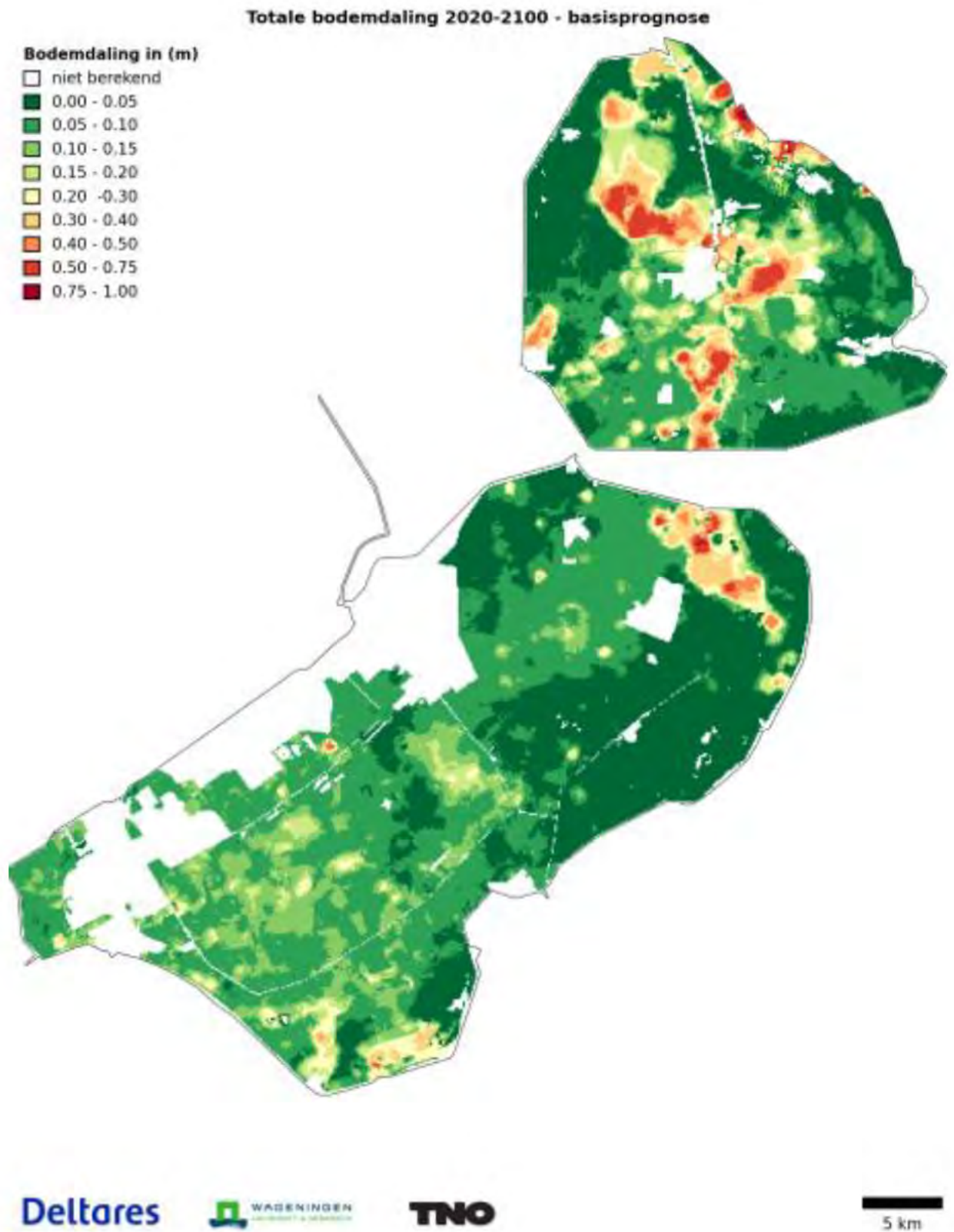
figuur 3-5 Bodemdaling prognose 2020 - 2100
