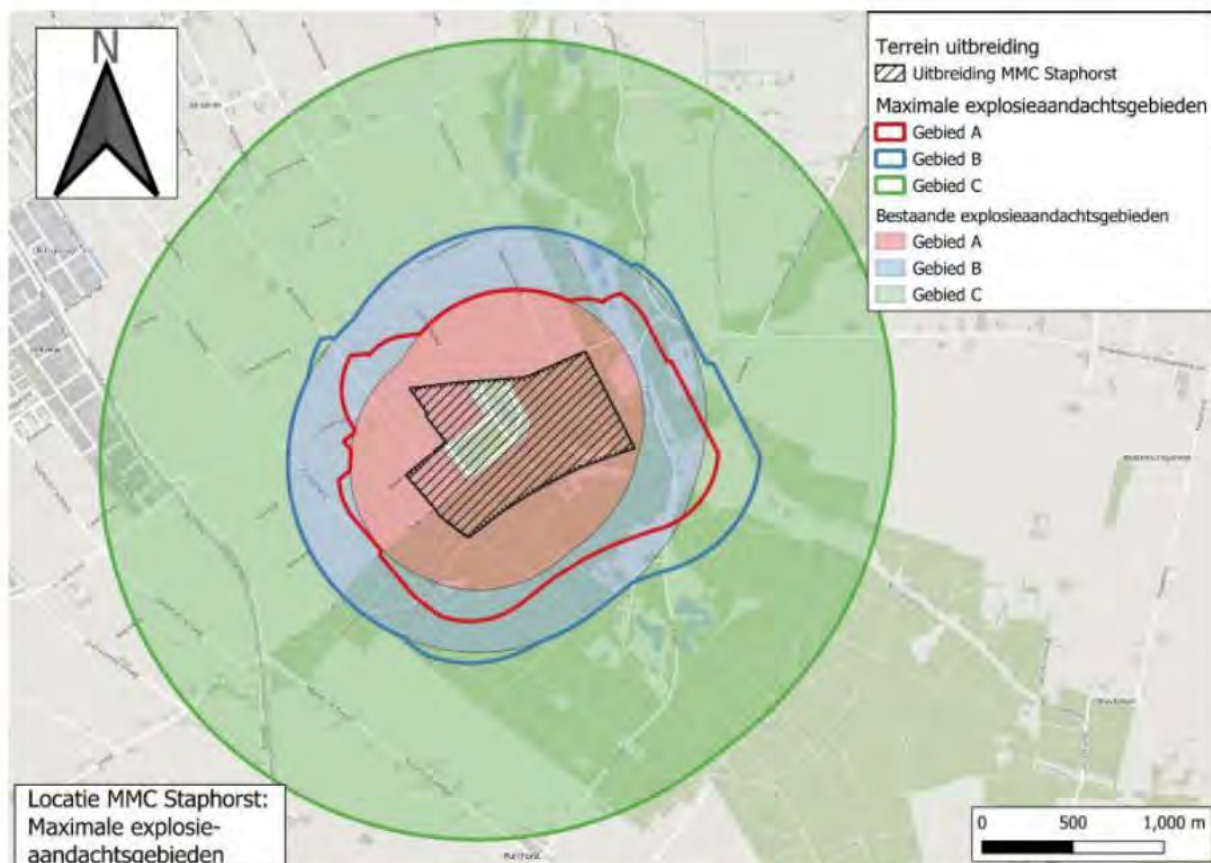
figuur 3-8 Overzicht van de militaire explosieaandachtsgebieden voor het maximale scenario.
