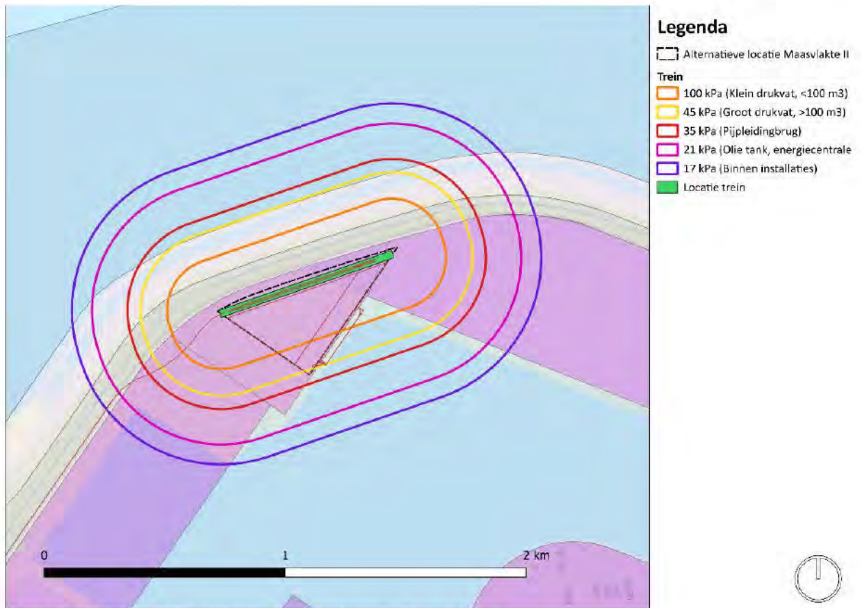
figuur 3-22 De ligging van de verschillende overdrukcontouren van de trein locatie
