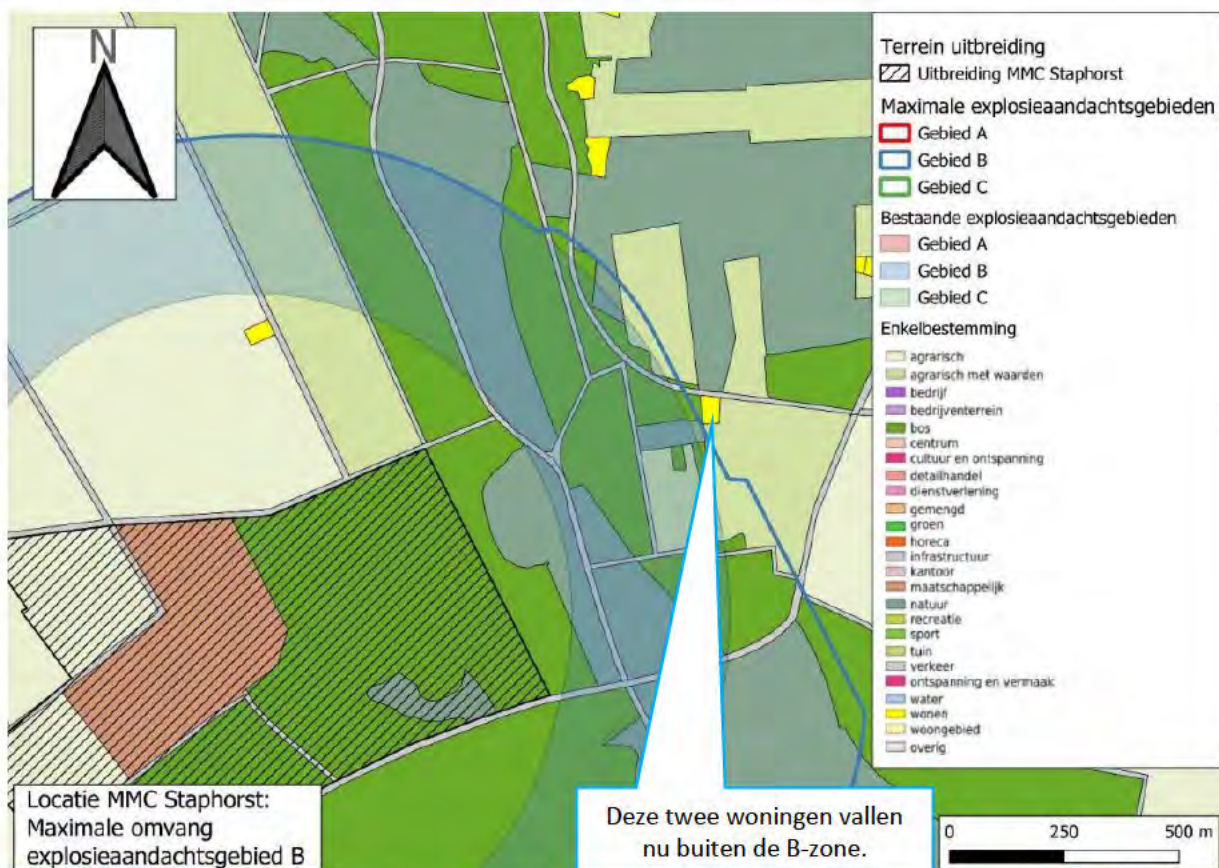
figuur 3-9 Maximale omvang van explosieaandachtsgebied B (B-zone) ingezoomd op de twee woningen die hier net buiten liggen aan de oostzijde van het nieuwe munitiecomplex.
