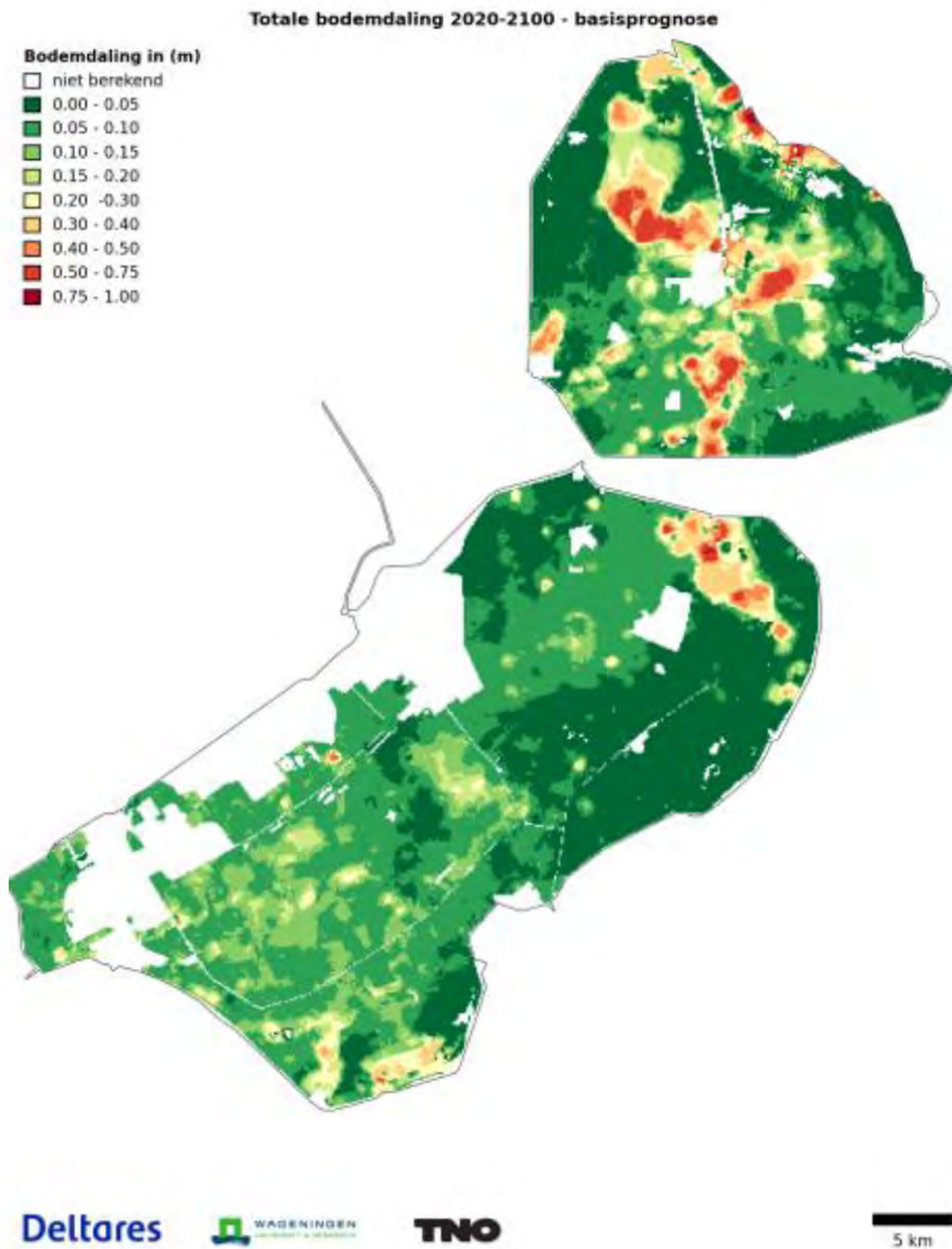
figuur 3-5 Bodemdaling prognose 2020 - 2100
